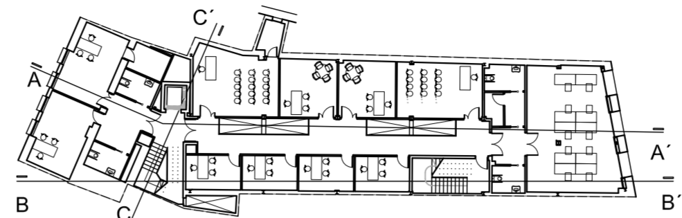
Planta primera
